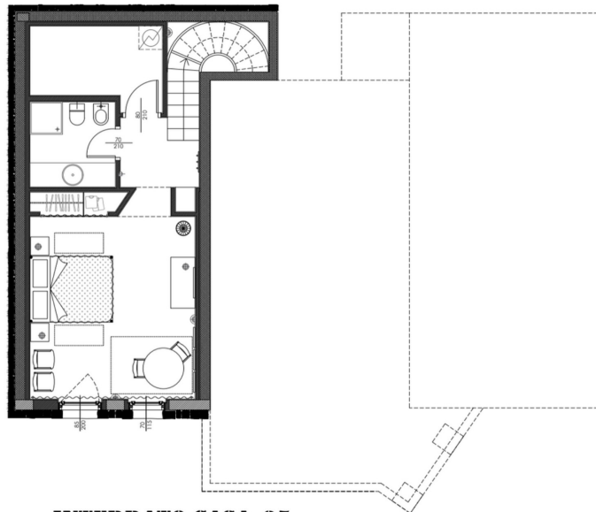
INTERRATO CASA 25
