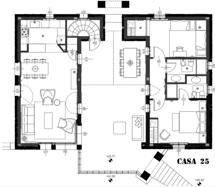
CASA 25 - Pianta piano terra 1:50 - arch. Laura Sonzogni_ ARREDO 20.03.2014
